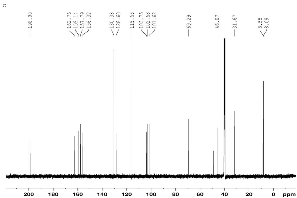
Fig 3. ^{13}\text{C} NMR
