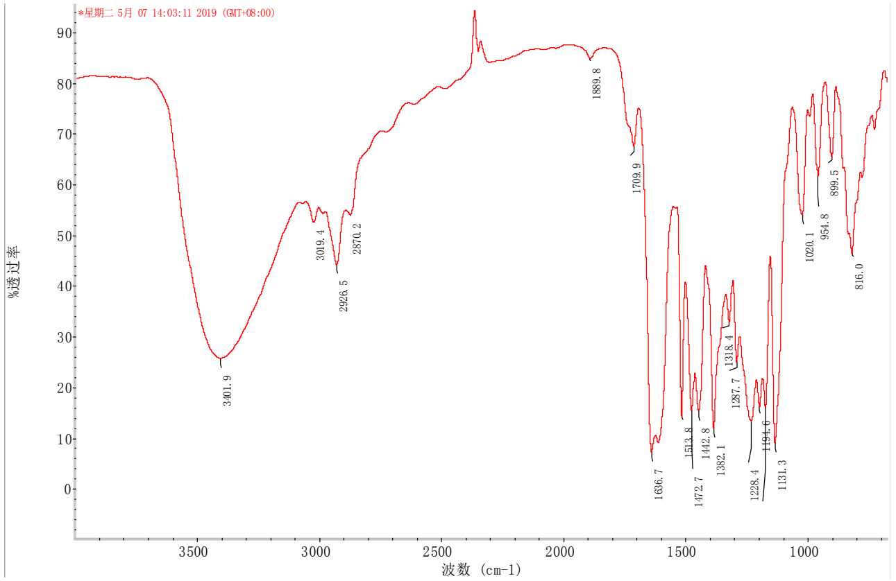
Fig 4. Micro IR
