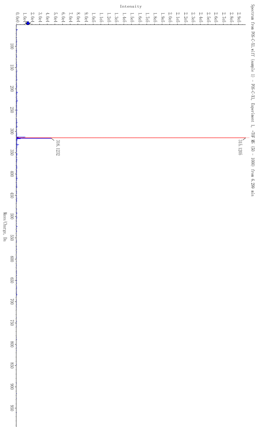
Fig 1. LC-HRMS
