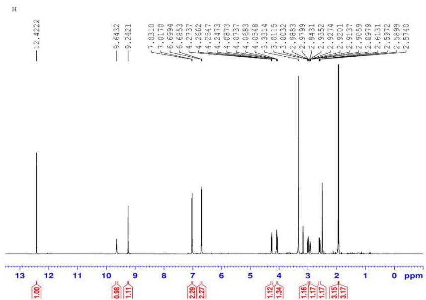
Fig 2. ^1\text{H} NMR
