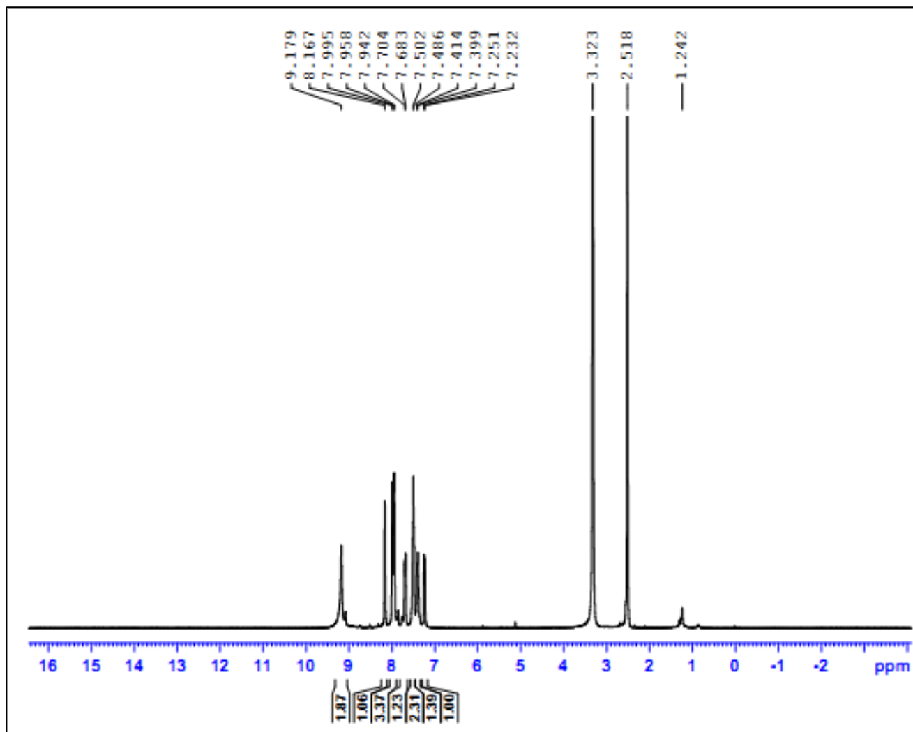
Fig.S12: ^1\text{H} NMR spectrum of 6-bromo-3-(4-phenyl-[1,2,3]triazol-1-yl)-chromen-2-ylideneamine 4g
