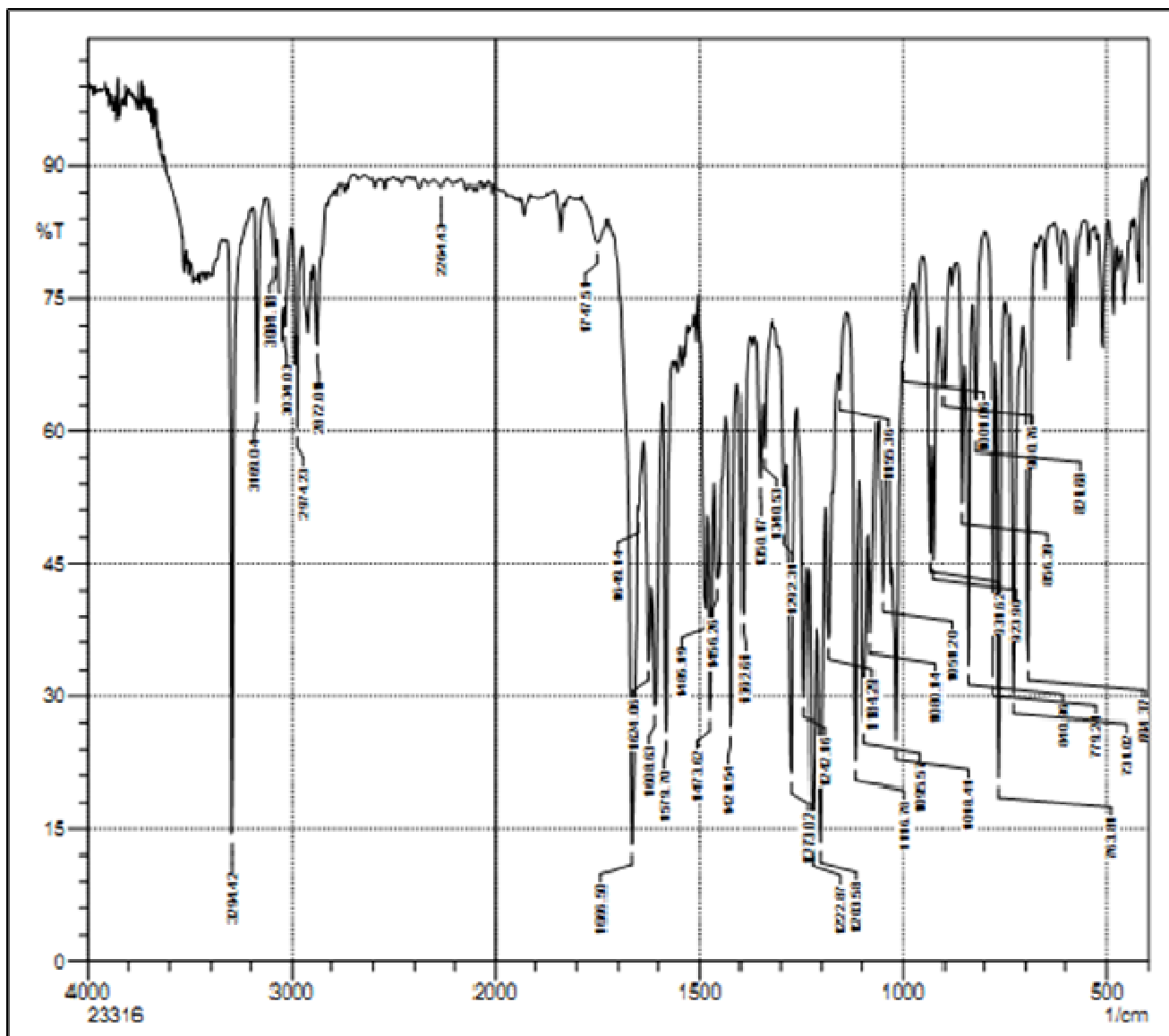
Fig.S8: IR spectrum of 8-Ethoxy-3-(4-phenyl-[1,2,3]triazol-1-yl)-chromen-2-ylideneamine 4c
