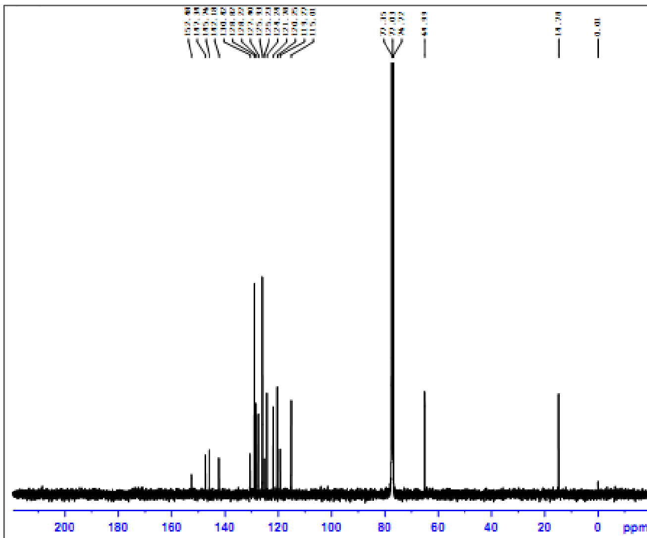
Fig.S7: ^{13}\text{C} NMR spectrum of 8-Ethoxy-3-(4-phenyl-[1,2,3]triazol-1-yl)-chromen-2-ylideneamine 4c
