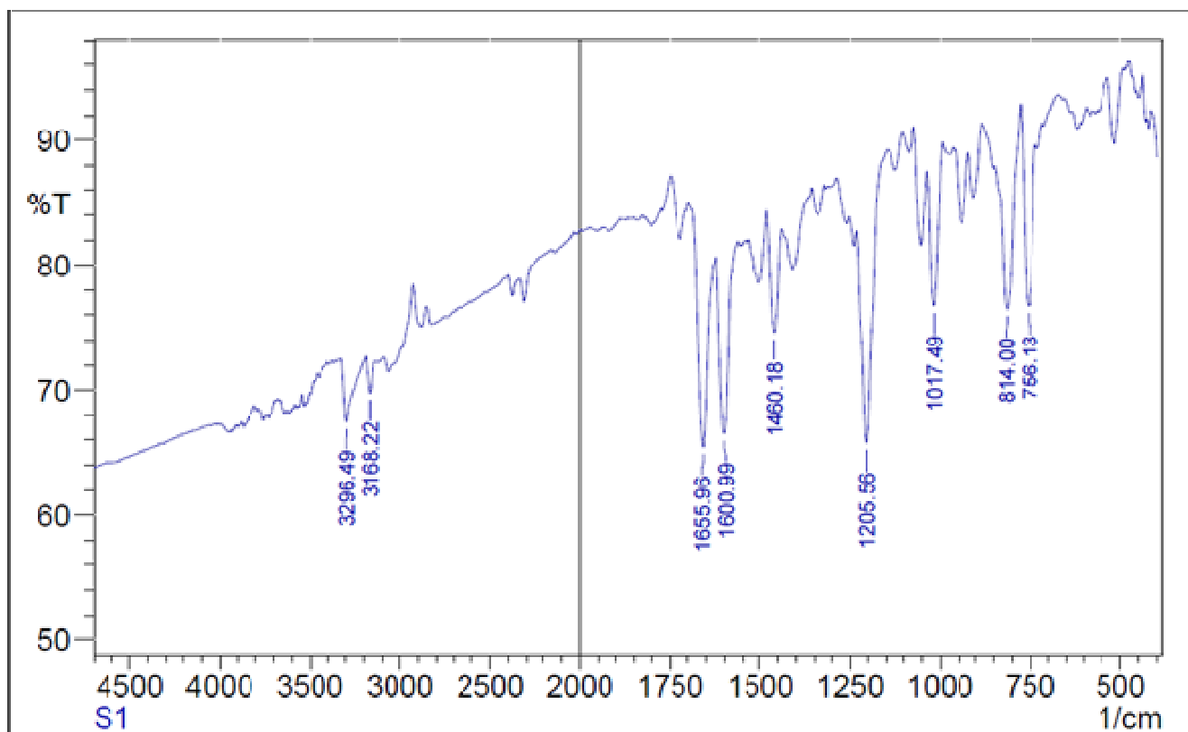
Fig.S5: IR spectrum of 3-(4-p-Tolyl-[1,2,3]triazol-1-yl)-chromen-2-ylideneamine 4b
