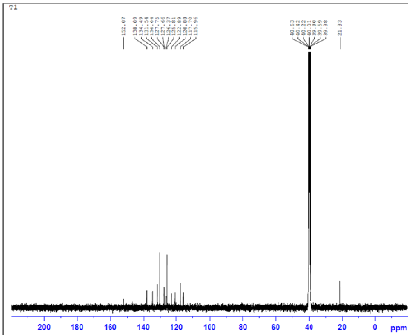
Fig.S15: ^{13}\text{C} NMR spectrum of 6-bromo-3-(4-p-tolyl-[1,2,3]triazol-1-yl)-chromen-2-ylideneamine 4h
