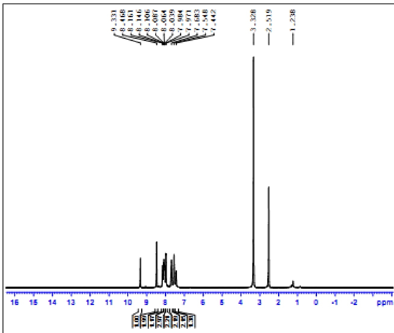
Fig.S1: 1 H NMR spectrum of 3-(4-Phenyl-[1,2,3]triazol-1-yl)-chromen-2-ylideneamine 4a
