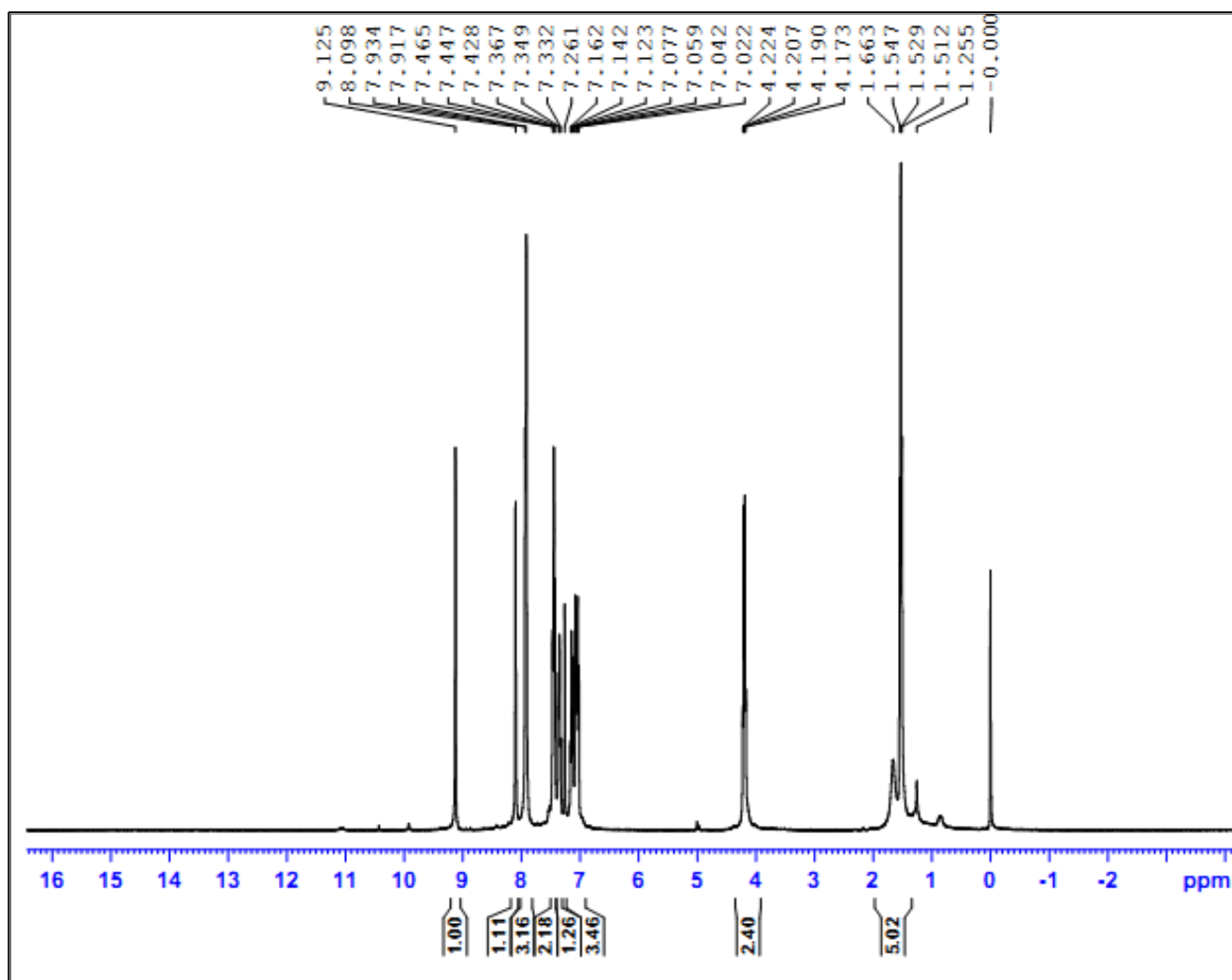
Fig.S6: ^1\text{H} NMR spectrum of 8-Ethoxy-3-(4-phenyl-[1,2,3]triazol-1-yl)-chromen-2-ylideneamine 4c
