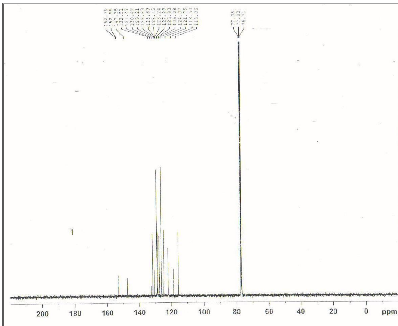
Fig.S2: ^{13}\text{C} NMR spectrum of 3-(4-Phenyl-[1,2,3]triazol-1-yl)-chromen-2-ylideneamine 4a
