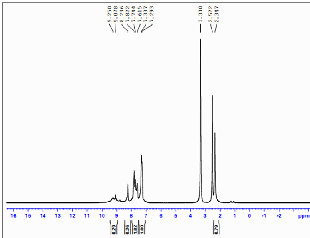
Fig.S4: 1 H NMR spectrum of 3-(4-p-Tolyl-[1,2,3]triazol-1-yl)-chromen-2-ylideneamine 4b
