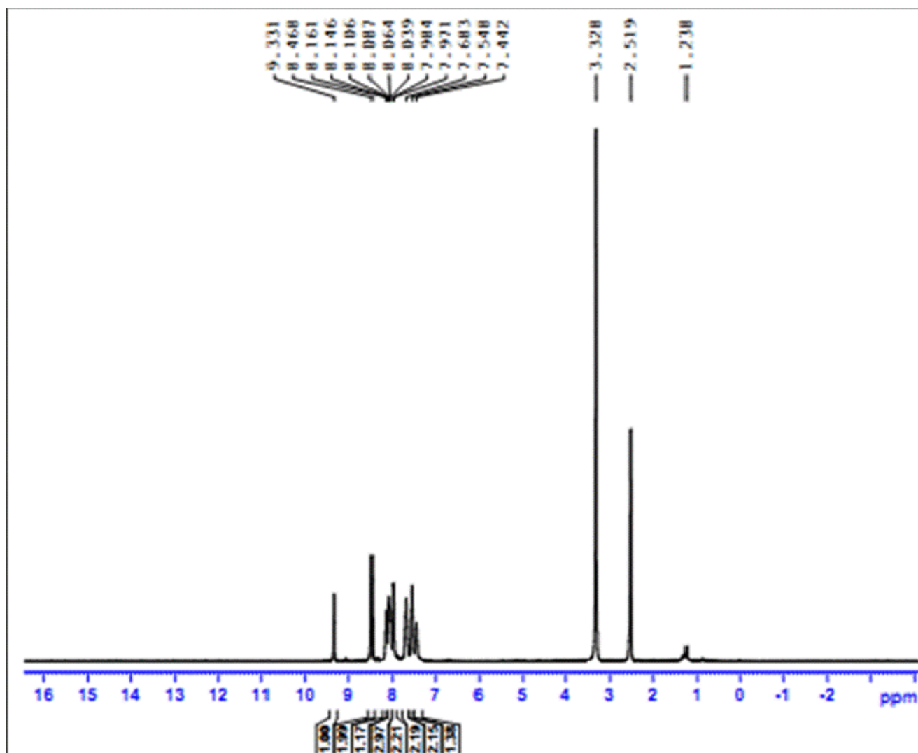
Fig.S16: ^1\text{H} NMR spectrum of 2-(4-Phenyl-[1,2,3]triazol-1-yl)-benzo[ f ]chromen-3-ylideneamine 6a
