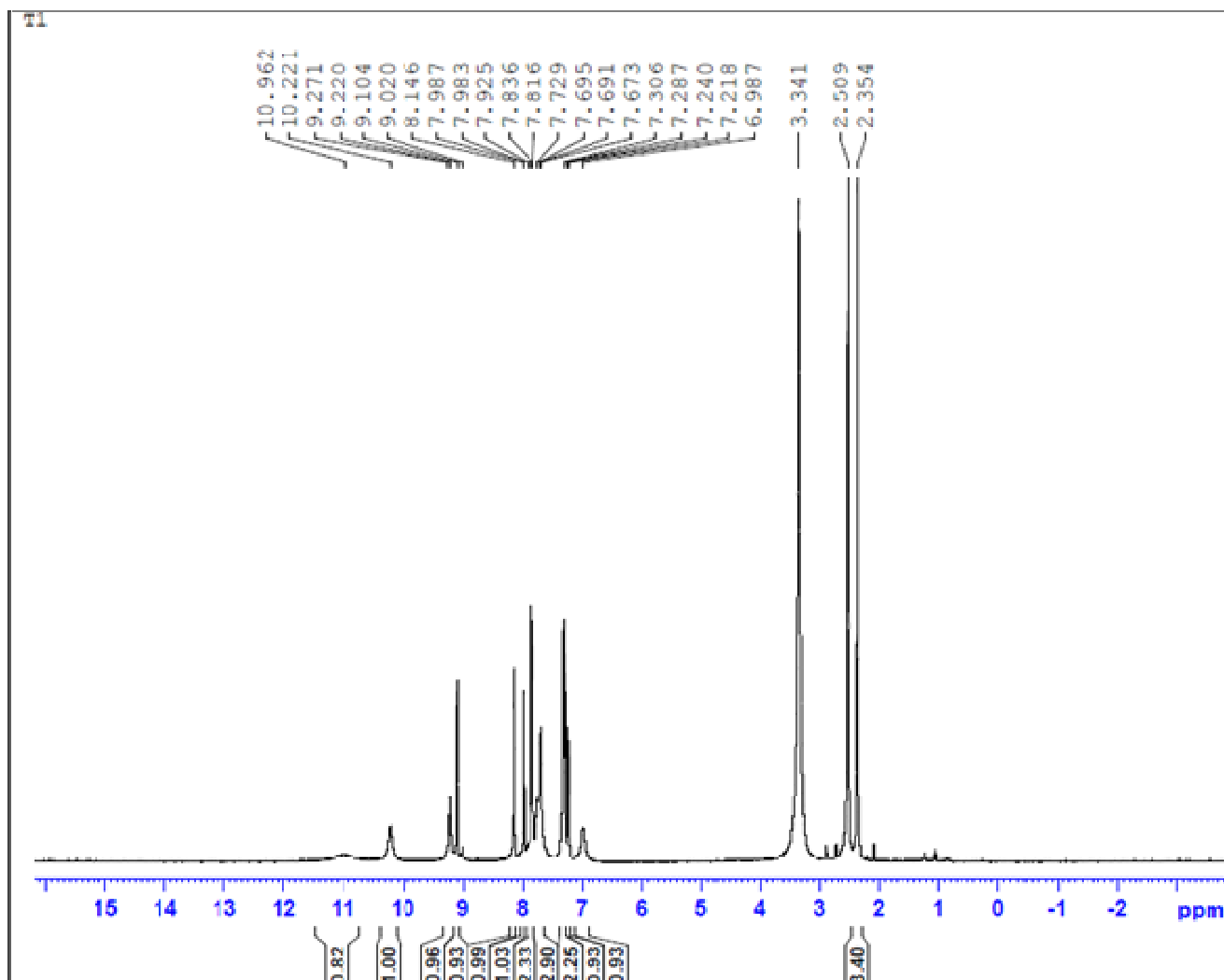
Fig.S14: 1 H NMR spectrum of 6-bromo-3-(4-p-tolyl-[1,2,3]triazol-1-yl)-chromen-2-ylideneamine 4h
