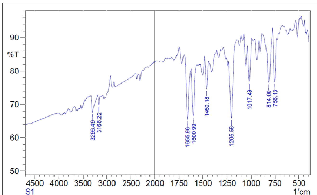
Fig.S10: IR spectrum of 8-Ethoxy-3-(4-p-tolyl-[1,2,3]triazol-1-yl)-chromen-2-ylideneamine 4d
