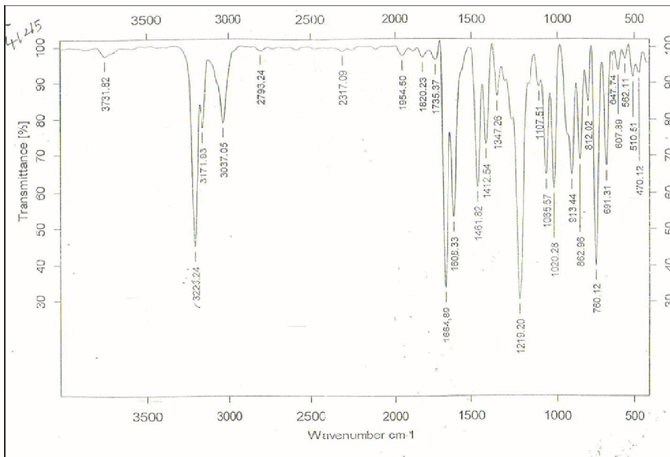
Fig.S3: IR spectrum of 3-(4-Phenyl-[1,2,3]triazol-1-yl)-chromen-2-ylideneamine 4a
