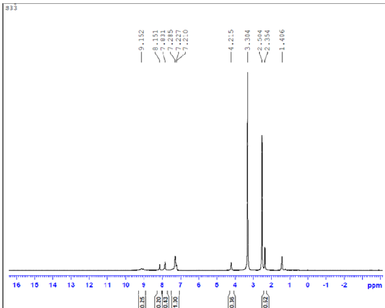
Fig.S9: 1 H NMR spectrum of 8-Ethoxy-3-(4-p-tolyl-[1,2,3]triazol-1-yl)-chromen-2-ylideneamine 4d
